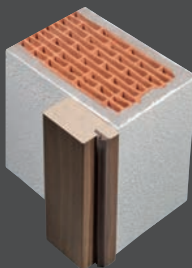
BLENDRAHMEN BM 45 auf der Wand, vor der Laibung montiert
